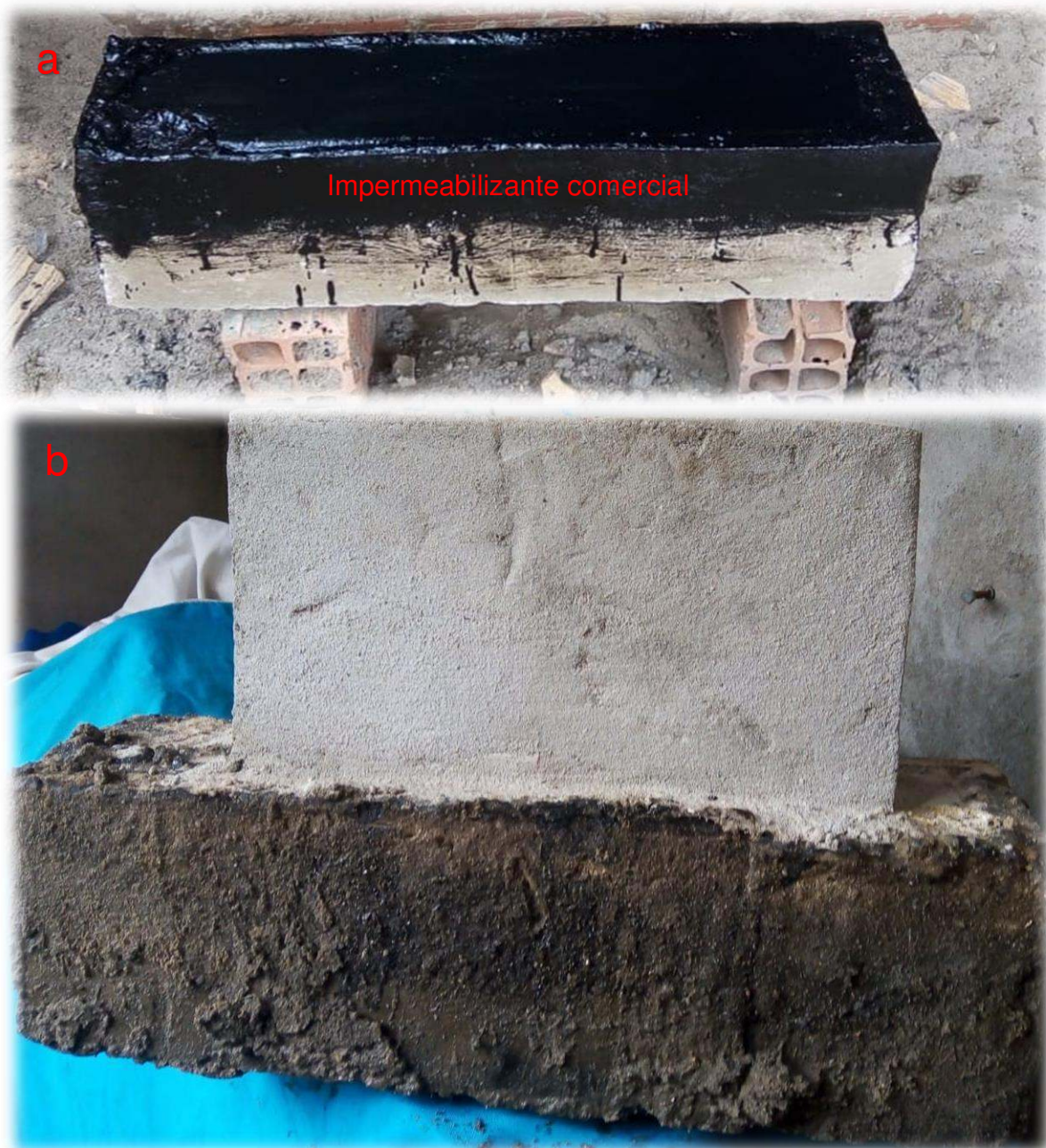
Figura 20 – a) viga impermeabilizada; b) viga atacada por ácido sulfúrico
