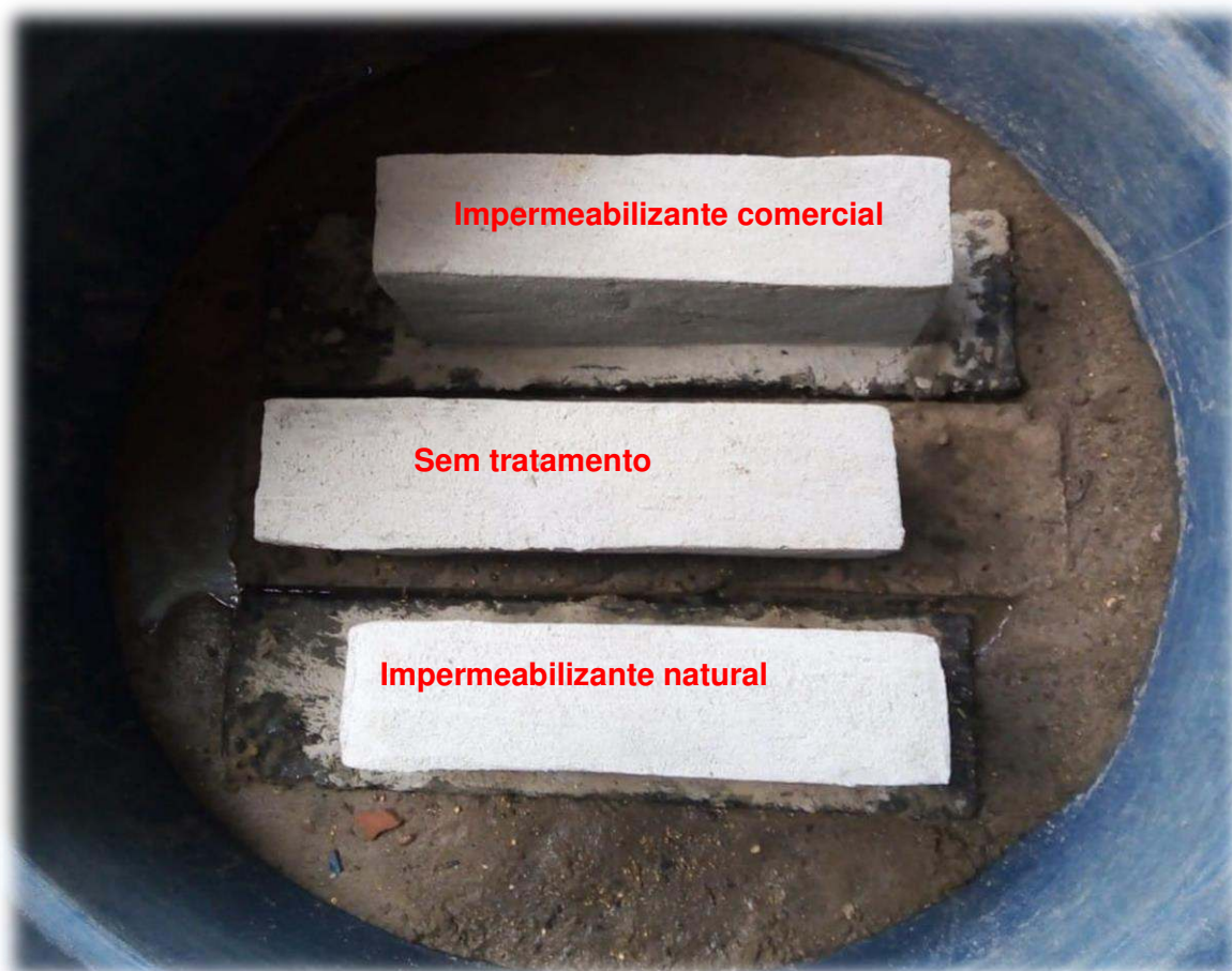
Figura 18 - Viga em local confinado
