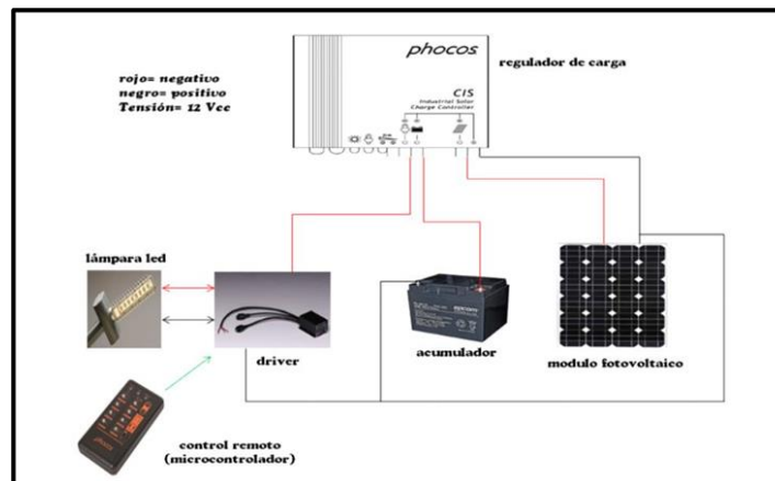
Figura 6: Esquema do circuito elétrico do sistema de iluminação fotovoltaica. Fonte: Soares (2012)
