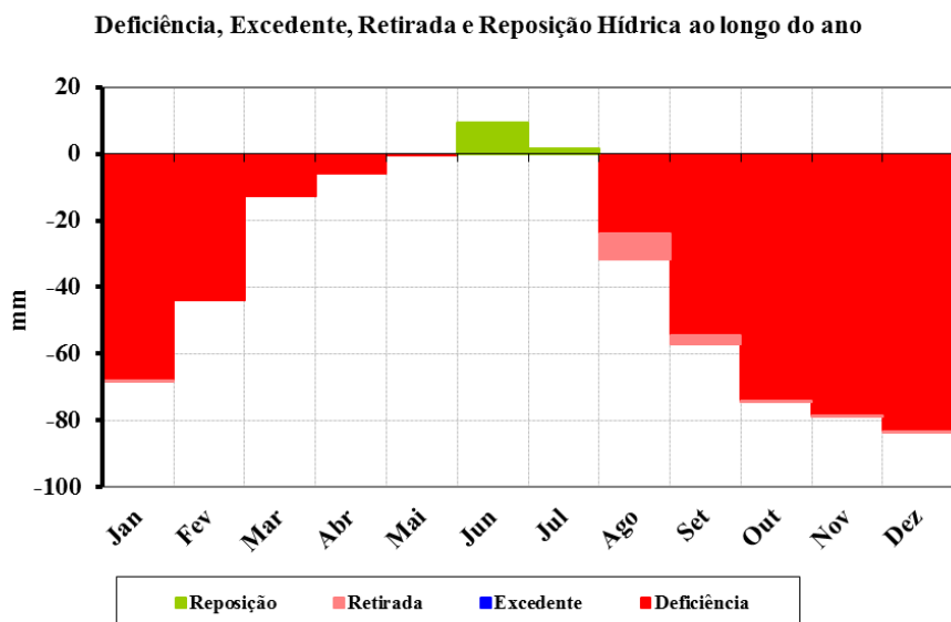
Figura 5. Balanço hídrico climatológico normal no período de 1920 a 2016 para o município de São Bento do Una para capacidade de campo de 25 mm. Fonte: Medeiros (2021).
