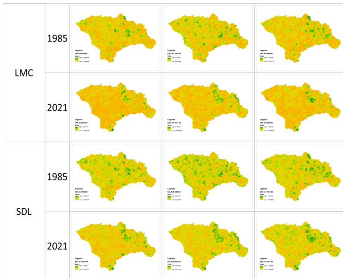
Figura 10. Mapas de complexidade das medidas LMC e SDL gerados pelo script CompPlex Janus a partir de imagens Landsat de 1985 e 2021 da microbacia hidrográfica do Córrego do Gregório (São Carlos - SP). OBS: Da esquerda para a direita, são apresentados os mapas gerados para as bandas 1, 2 e 3, respectivamente. Tons mais escuros de verde no mapa representam valores mais altos para a respectiva medida, enquanto os valores mais baixos são representados pelos tons mais claros de laranja.
