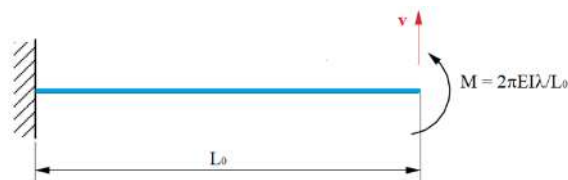
Figura 5 - Modelo estrutural da viga em balanço.
