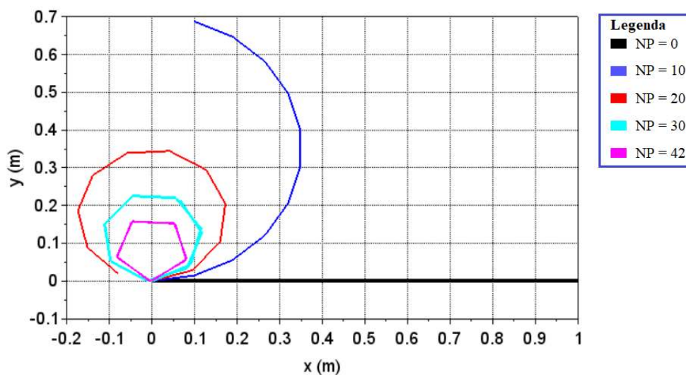
Figura 7 - Configurações deformadas da viga.
