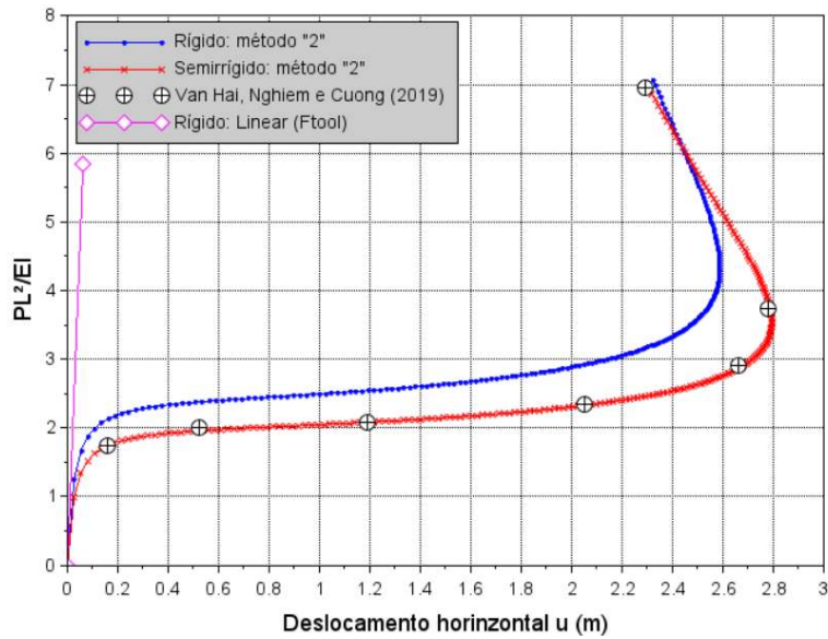
Figura 3 - Trajetória de equilíbrio da coluna.
