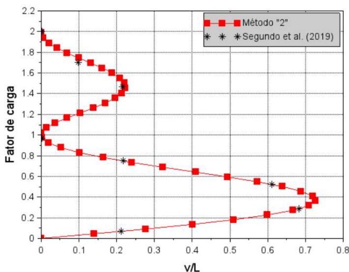
Figura 6 - Trajetória de equilíbrio da viga.
