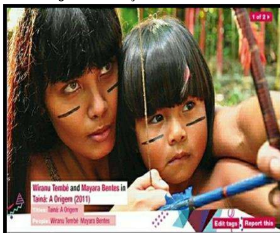
Imagem 4 - Reação Não-Transacional
