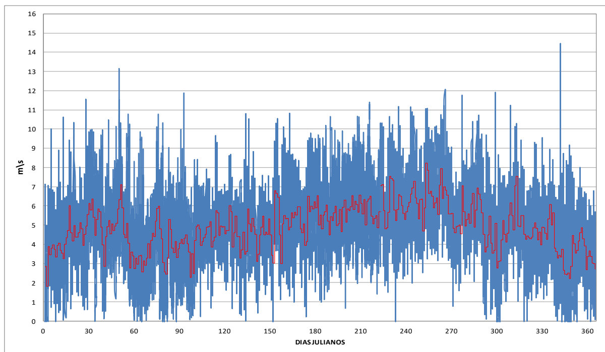
Figura 4: Variação anual dos ventos a 50 metros.
