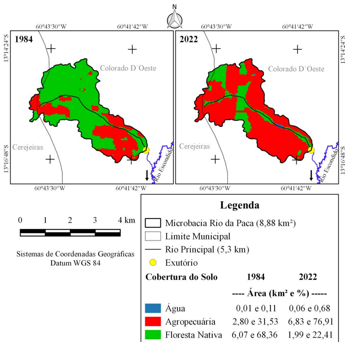
Figura 6. Dinâmica da cobertura do solo na microbacia Rio da Paca, Amazônia Ocidental, Brasil
