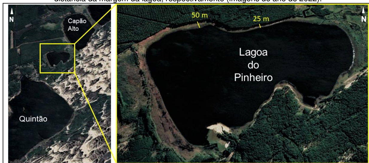
Figura 8 – Imagem da Lagoa 9 – Pinheiro, exibindo as APPs completamente invadidas pela silvicultura. Na porção superior da imagem, espécimes de Pinus plantadas à 50 e 25 metros de distância da margem da lagoa, respectivamente (imagens do ano de 2022).
