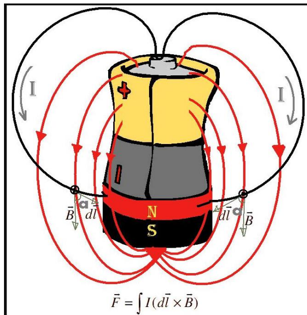
Figura 4: Campo magnético de um motor homopolar. O campo magnético se estende até a bateria por causa de seu invólucro metálico
