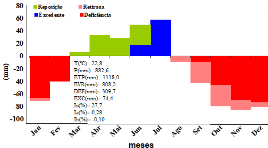
Figura 2. Gráfico do balanço hídrico no período de 1962 a 2019 para a bacia hidrográfica do rio Ipojuca - PE.
