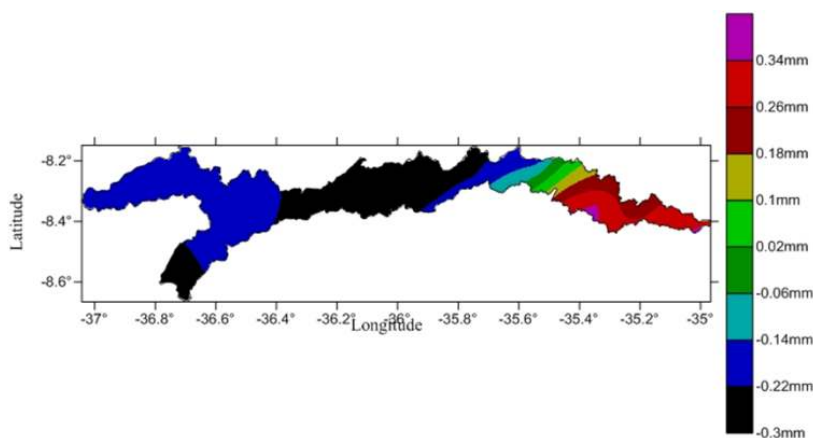
Figura 6. Índice hídrico (%) do período de 1962 a 2019 para a bacia hidrográfica do rio Ipojuca - PE.
