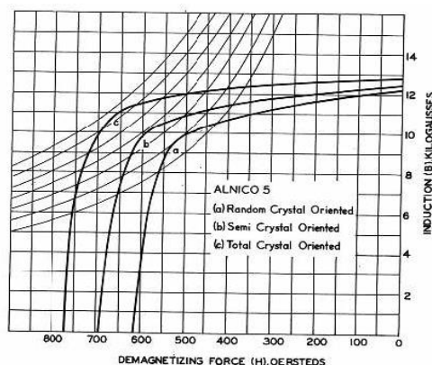
Figura 1: Curvas de desmagnetização para imãs de AlNiCo 5 (Parker, Studders).
