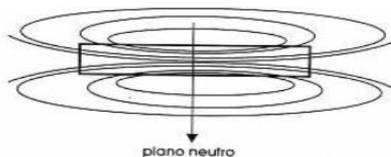
Figura 2: Linhas de indução em uma barra magnetizada (Faria, Lima).
