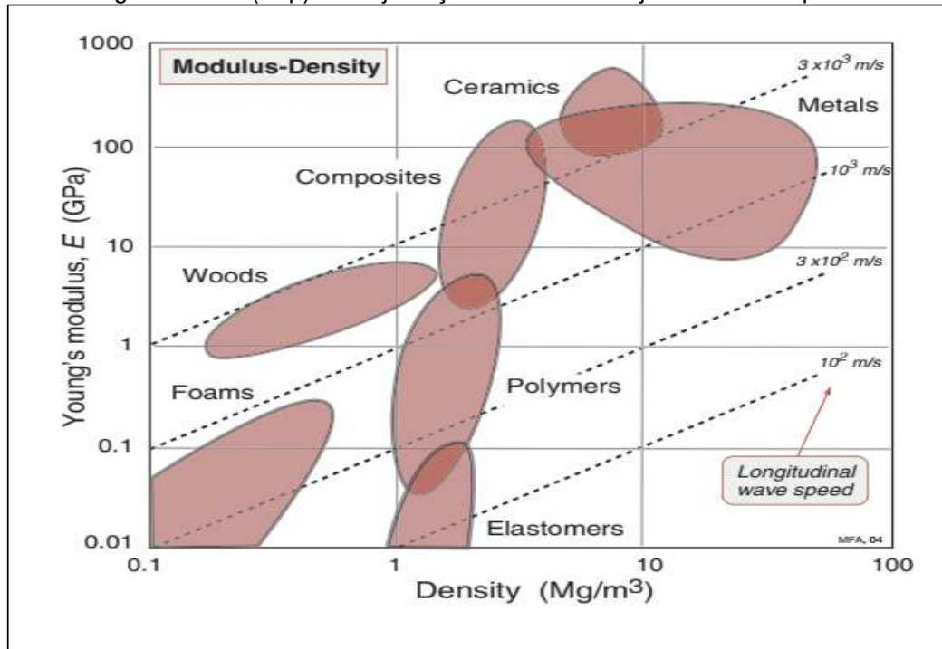
Figura 1: A ideia de um gráfico de propriedades de materiais: o módulo de Young, E, é plotado em relação à densidade, em escalas logarítmicas. Cada classe de material ocupa uma parte característica do gráfico. As escalas logarítmicas permitem que a velocidade da onda elástica longitudinal v = (E/\rho)^{1/2} seja traçada como um conjunto de linhas paralelas.
