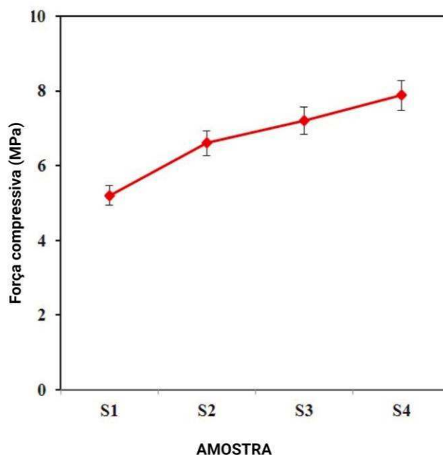
Figura 11 - Resultados de resistência à compressão de amostras de bio-nanocompósitos porosos contendo várias quantidades de nanopartículas magnéticas. Fonte: (34)
