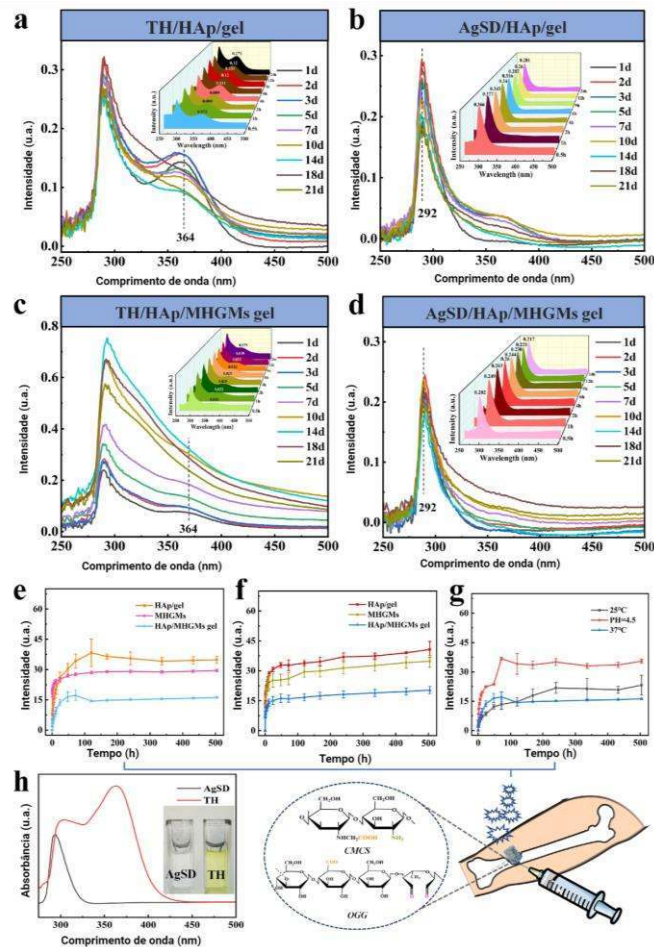
Figura 18 - Curvas de absorção UV-vis de TH (a) e AgSD (b) liberados por HAp/gel em diferentes momentos. Curvas de absorção UV-vis de TH (c) e AgSD (d) liberados pelo gel de HAp/MHGMs em diferentes momentos. Liberação cumulativa de TH (e) e AgSD (f) de HAp/gel, MHGMs e HAp/MHGMs gel em PBS a 37°C. (g) Liberação cumulativa de TH do gel HAp/MHGMs em diferentes ambientes. (h) Os espectros UV-vis do AgSD e TH. Os valores relatados são uma média de n = 3 , \pm desvio padrão. Fonte: (37).
