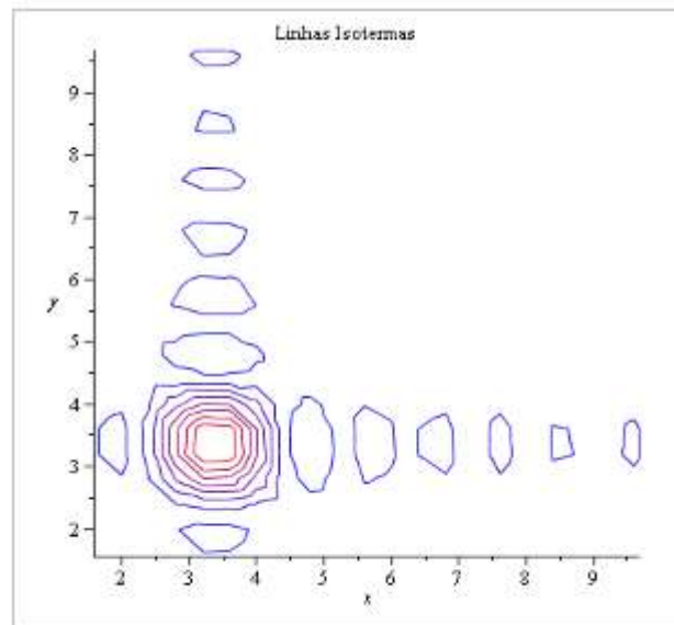
Figura 4 b: Análise feita mostra a distribuição de temperatura ao longo de toda a superfície do chip no tempo
