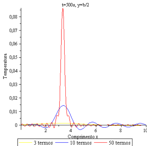
Figura 3: Influência do número de termos na distribuição de temperatura da placa.
