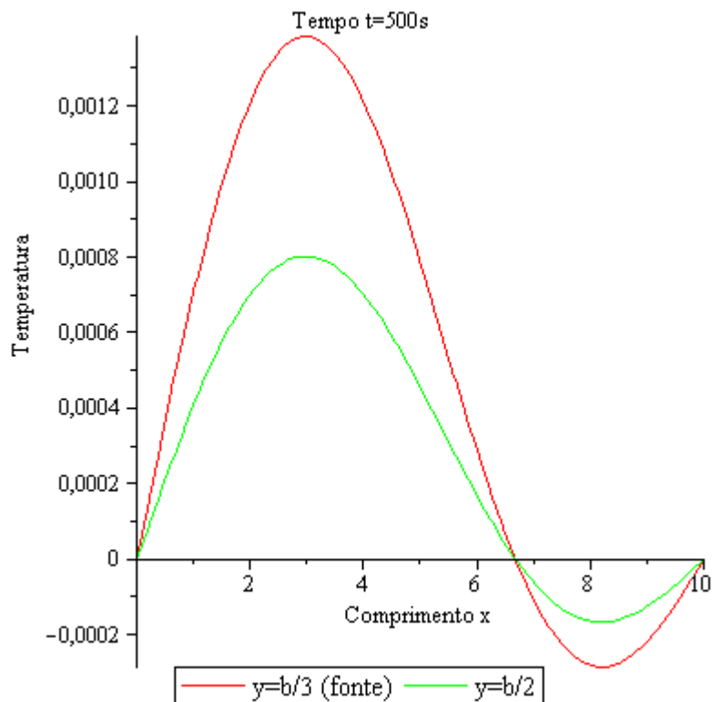
Figura 2: Influência da proximidade da fonte de calor na temperatura da placa.
