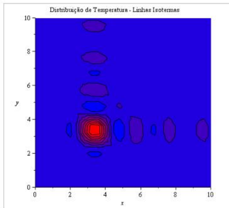
Figura 4 a: Análise feita mostra a distribuição de temperatura ao longo de toda a superfície do chip no tempo
