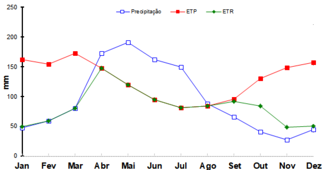
Figura 2. Gráfico do balanço hídrico referente à precipitação; evapotranspiração potencial e evaporação real do período (1964-2020) em Amparo de São Francisco – SE. Fonte: França (2021).
