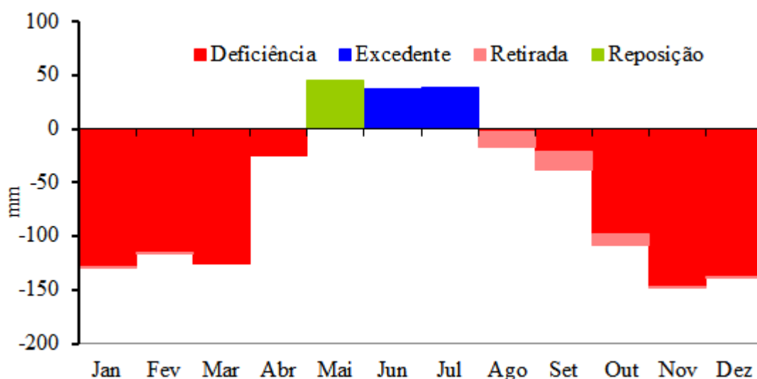
Figura 3. Gráfico do balanço referente à deficiência, excedente, retirada e reposição d'água 2070-2099 para Amparo de São Francisco – SE. Fonte: França (2021).
