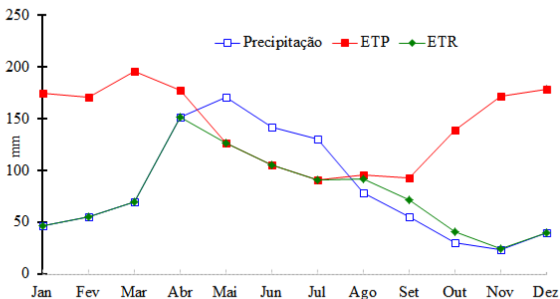
Figura 4. Gráfico do balanço hídrico referente à precipitação; evapotranspiração potencial e evaporação real do período (2070-2099) em Amparo de São Francisco – SE. Fonte: França (2021).
