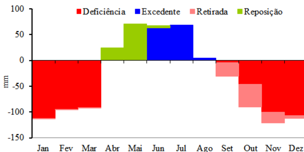
Figura 1. Gráfico do balanço referente à deficiência, excedente, retirada e reposição d'água 1964-2020 para Amparo de São Francisco – SE.
