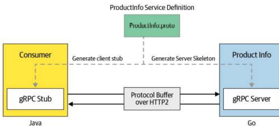
Figura 2 - Esquema exemplificando o funcionamento de uma chamada gRPC. Fonte: INDRASIRI; KURUPPU. (2020, p. 40)
