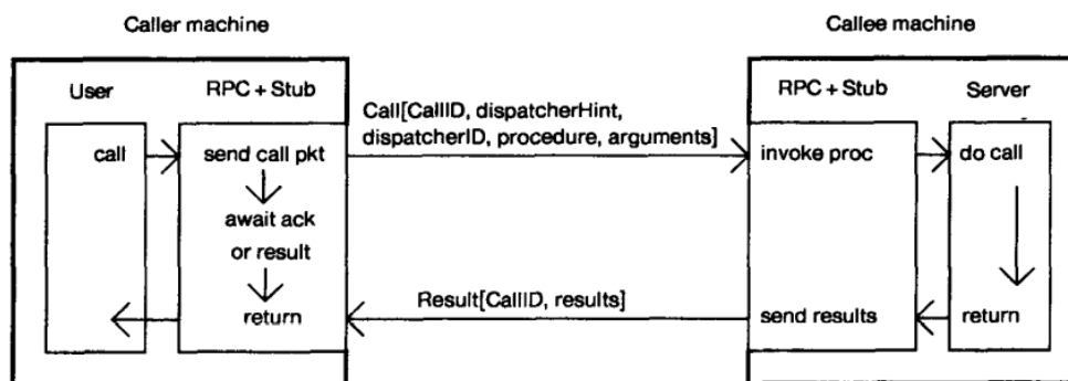
Figura 1 - Esquema exemplificando o funcionamento de uma chamada RPC Fonte: BIRRELL; NELSON. (1984, p. 39)
