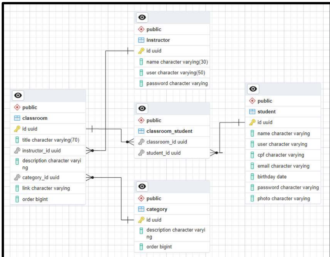
Figura 3. Diagrama Entidade-Relacionamento
