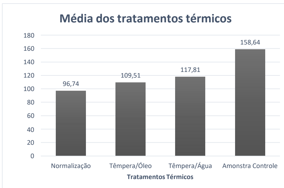
Figura 6: Gráfico média dos tratamentos térmicos
