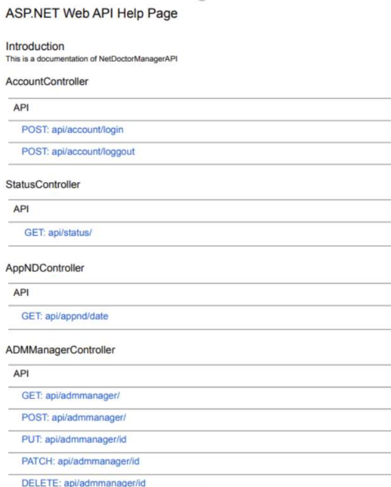
Figura 9 – Implementação da Web API Restful (configuração)
