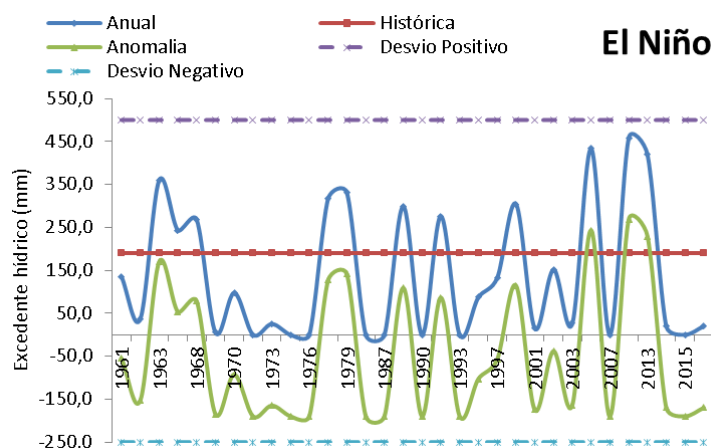
Figura 8. Variação do excedente hídrico em anos de El Niño em Bom Jesus-PI.
