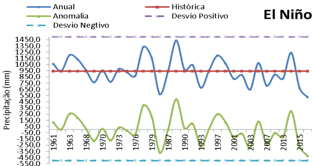
Figura 2. Variação da precipitação em anos de El Niño em Bom Jesus, Piauí.
