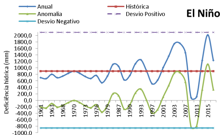
Figura 6. Variação da deficiência hídrica em anos de El Niño em Bom Jesus, Piauí.
