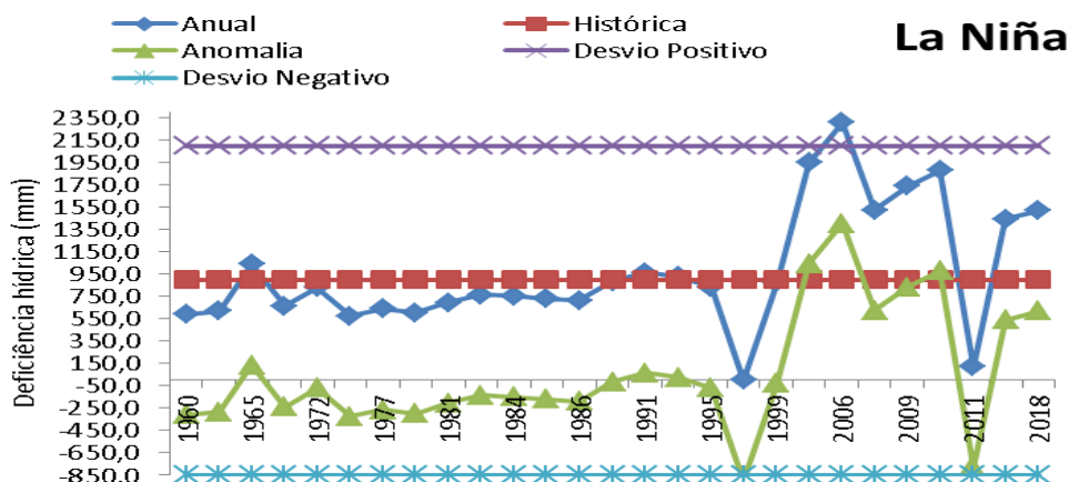
Figura 7. Variação da deficiência hídrica em anos e La Niña em Bom Jesus, Piauí.
