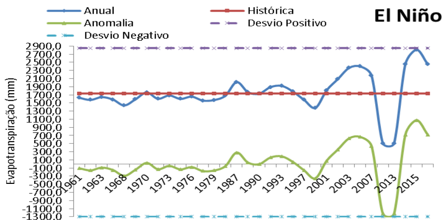
Figura 4. Variação da evapotranspiração em anos de El Niño em Bom Jesus, Piauí.
