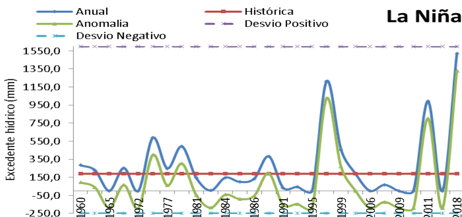
Figura 9. Variação do excedente hídrico em anos de La Niña em Bom Jesus, Piauí.
