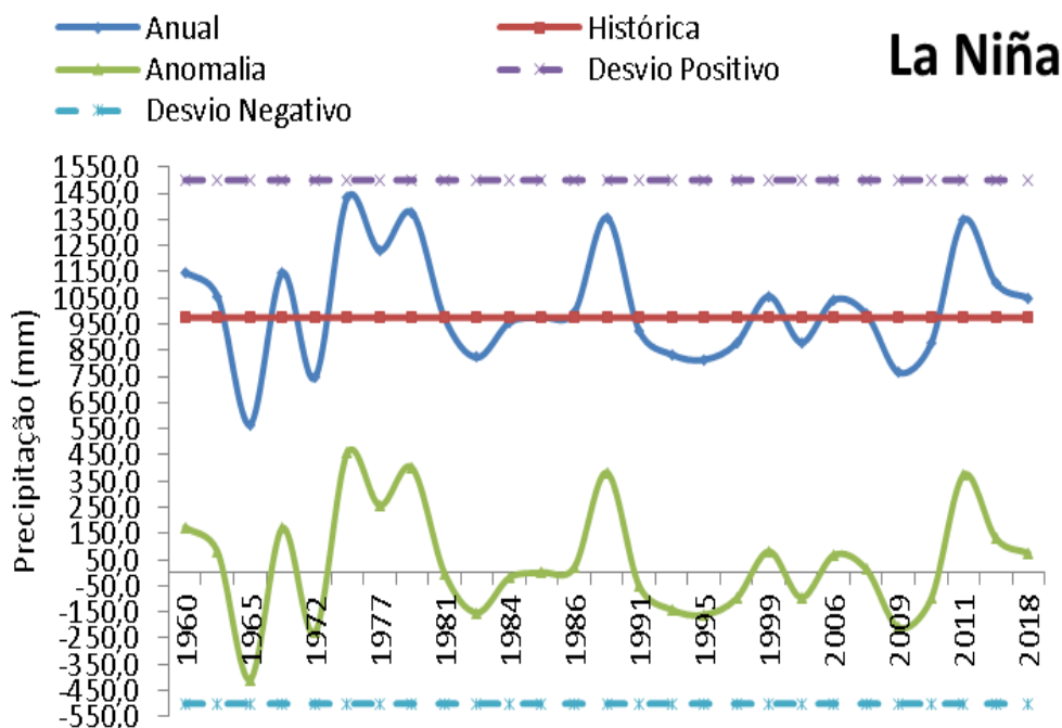
Figura 3. Variação da precipitação em anos de La Niña em Bom Jesus, Piauí.
