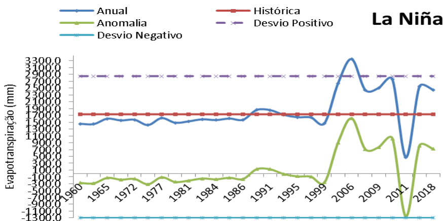
Figura 5. Variação da evapotranspiração em anos e La Niña em Bom Jesus-PI.
