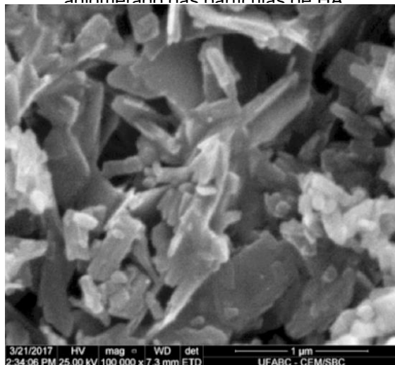
Figura 1: Micrografia obtida por microscopia eletrônica de varredura ilustrando o aspecto lamelar e aglomerado das partículas de HA
