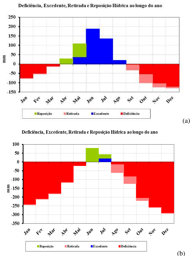
Figura 6. Gráficos do Balanço Hídrico climatológico da área da unidade Acadêmica do Cabo de Santo Agostinho (UACSA) com Capacidade de água disponível (CAD) de 100 mm e com aumento de 1°C na temperatura e redução de 10% na precipitação (a) e com aumento de 4°C na temperatura e redução de 20% na precipitação (b). FONTE: Medeiros (2021).
