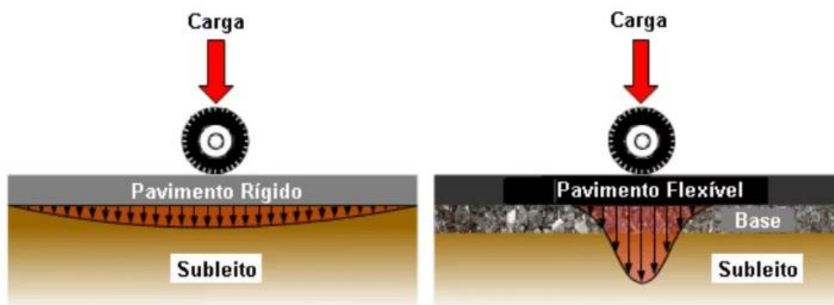
Figura 6: Deformação pela carga nos pavimentos
