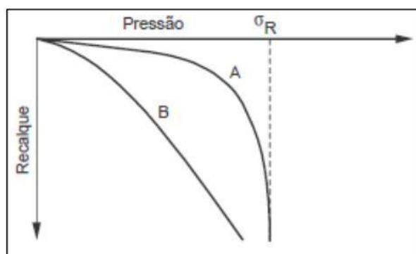
Figura 1- Curvas pressões x recalques
