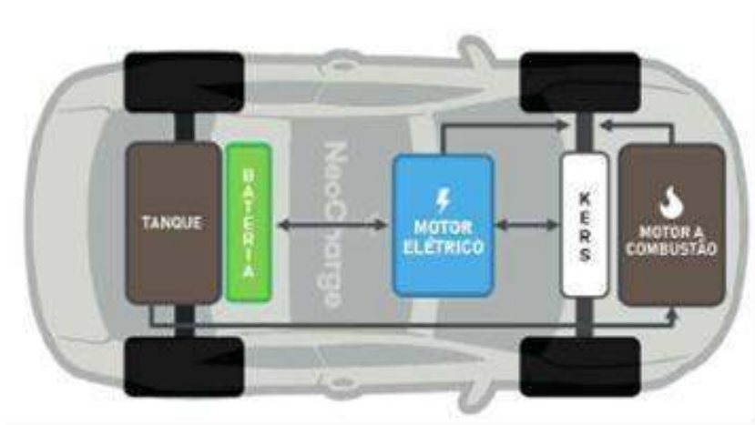
Figura 3: Esquema de funcionamento de um HEV Fonte: Adaptado de Neocharge (2021 apud SILVA, 2023, p.16)
